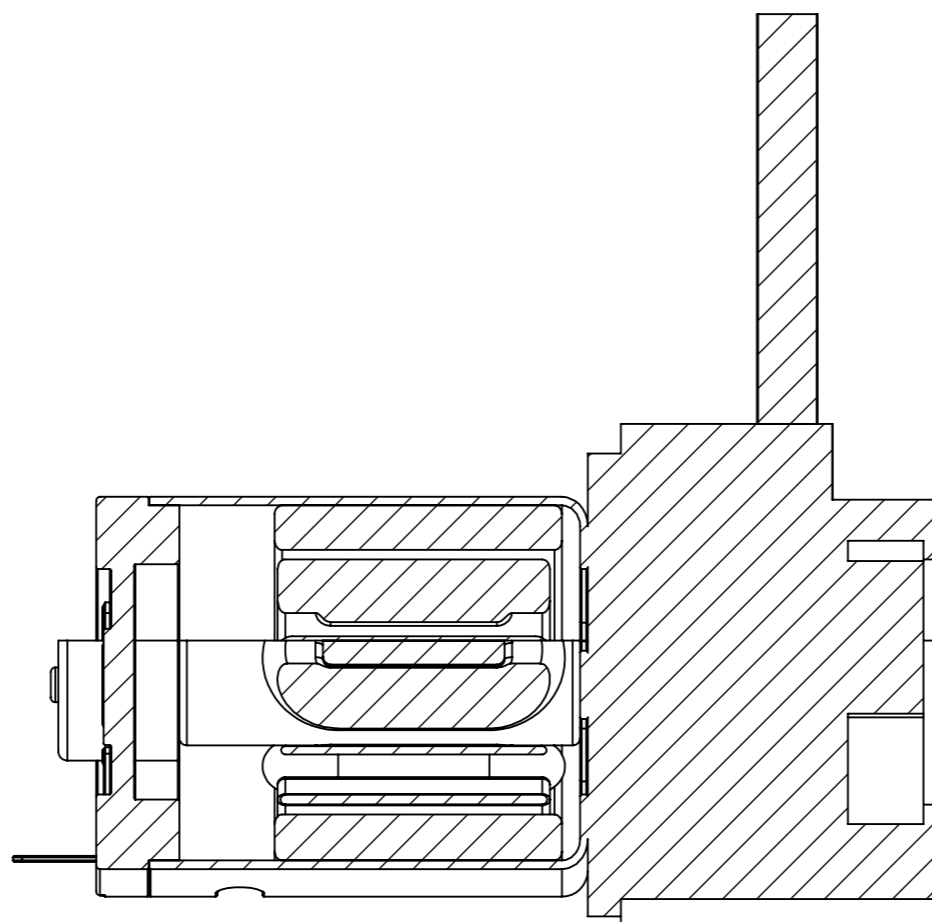
SEÇÃO A-A
